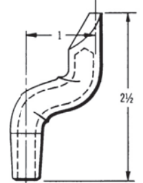
FD-1428-16 FA-2428-16
